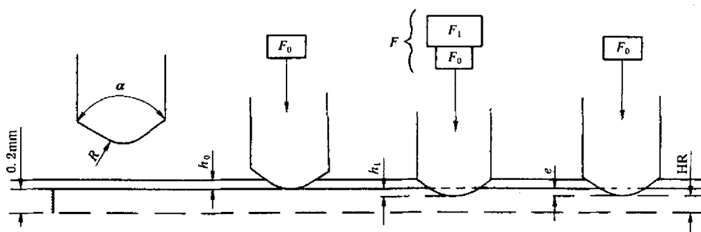
图1 HRC、HRA 试验示意图
