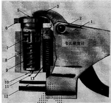
1—框架；2—支撑轴；3—下手柄；4—复位键；5—调节螺钉；6—测量指示装置； 7—调节螺母；8—压针筒；9—施力弹簧；10—限位；11—压针；12—砧座；13—复位弹簧
