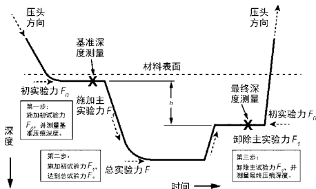
图 1 洛氏硬度试验方法 (示意图)
