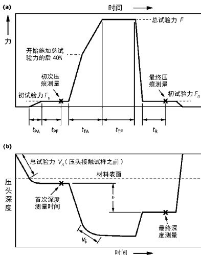
图 2 (a).力-时间示意图; (b)压头深度-时间示意图 (HRC 测试举例说明测试周期)
