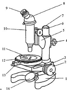
图4 测量显微镜外形图
