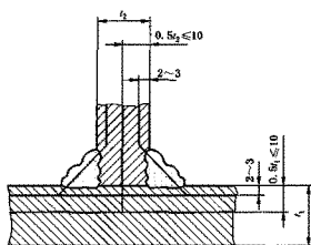
g) 双面角焊缝(多道)
