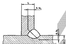
c) 单面角焊缝(单道)
