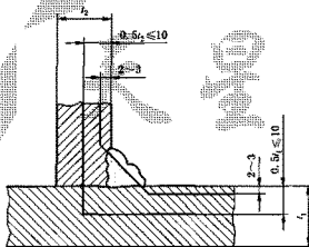
f) 单面角焊缝(多道)
