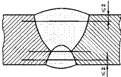
b) 双面焊对接焊缝
