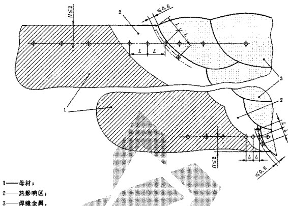
图7 钢板部多道焊缝评估硬化程度的测点位置示意图
