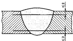
a) 单面焊对接焊缝
