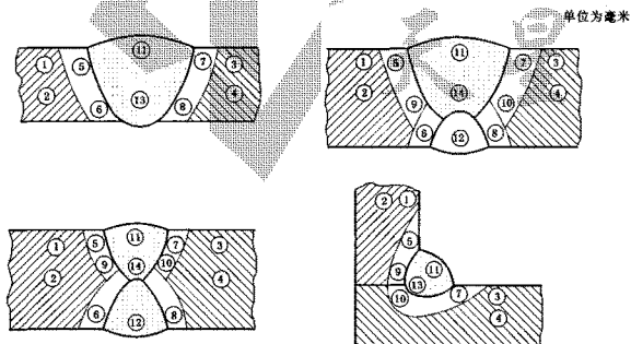
图7 钢板部多道焊缝评估硬化程度的测点位置示意图
