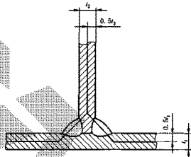
d) 双面角焊缝(单道)
