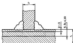
h) 双面角焊缝(多道, 肋板不承载)
